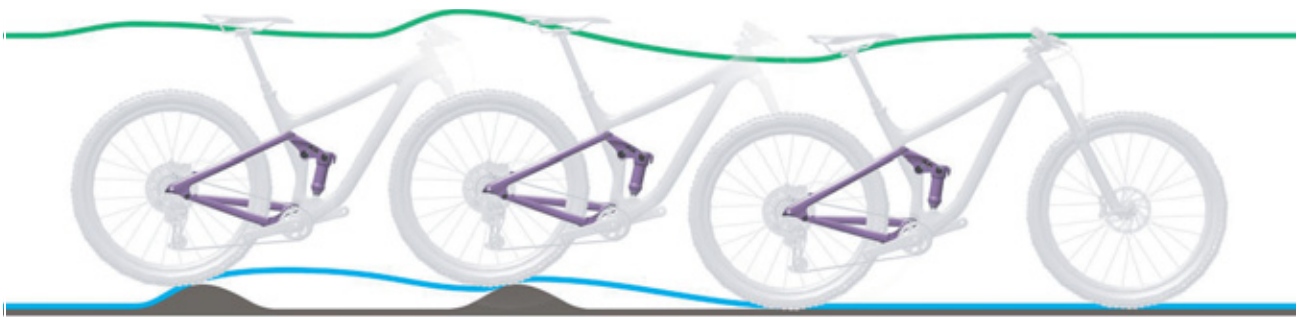
Figura 212: Descompresión demasiado lenta del amortiguador de la horquilla trasera
