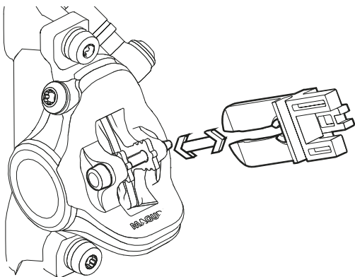
Figura 37: Fijación del seguro de transporte
