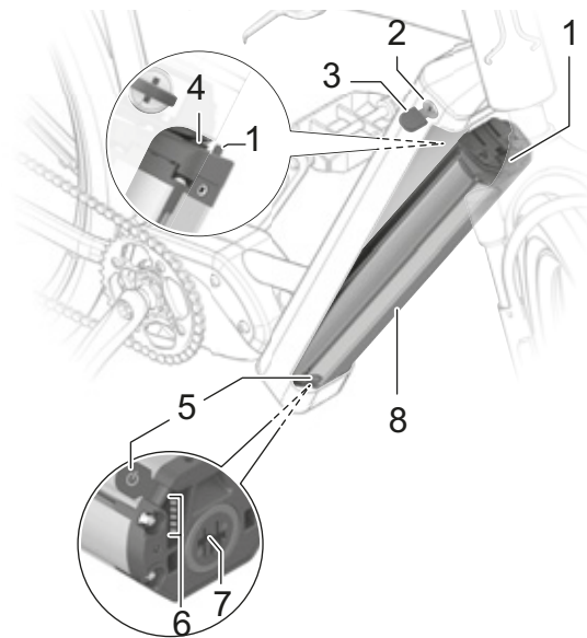
Figura 29: Detalle de la PowerTube 750
