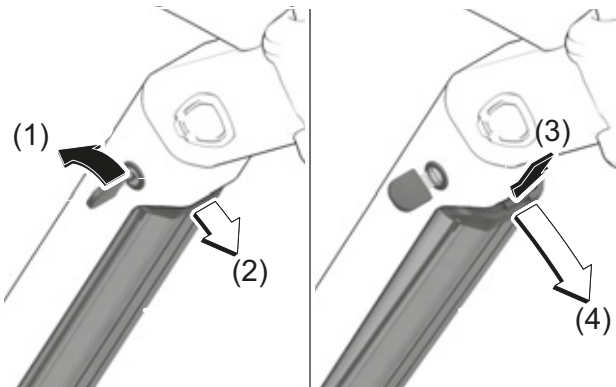
Figura 101: Extracción de la batería integrada
