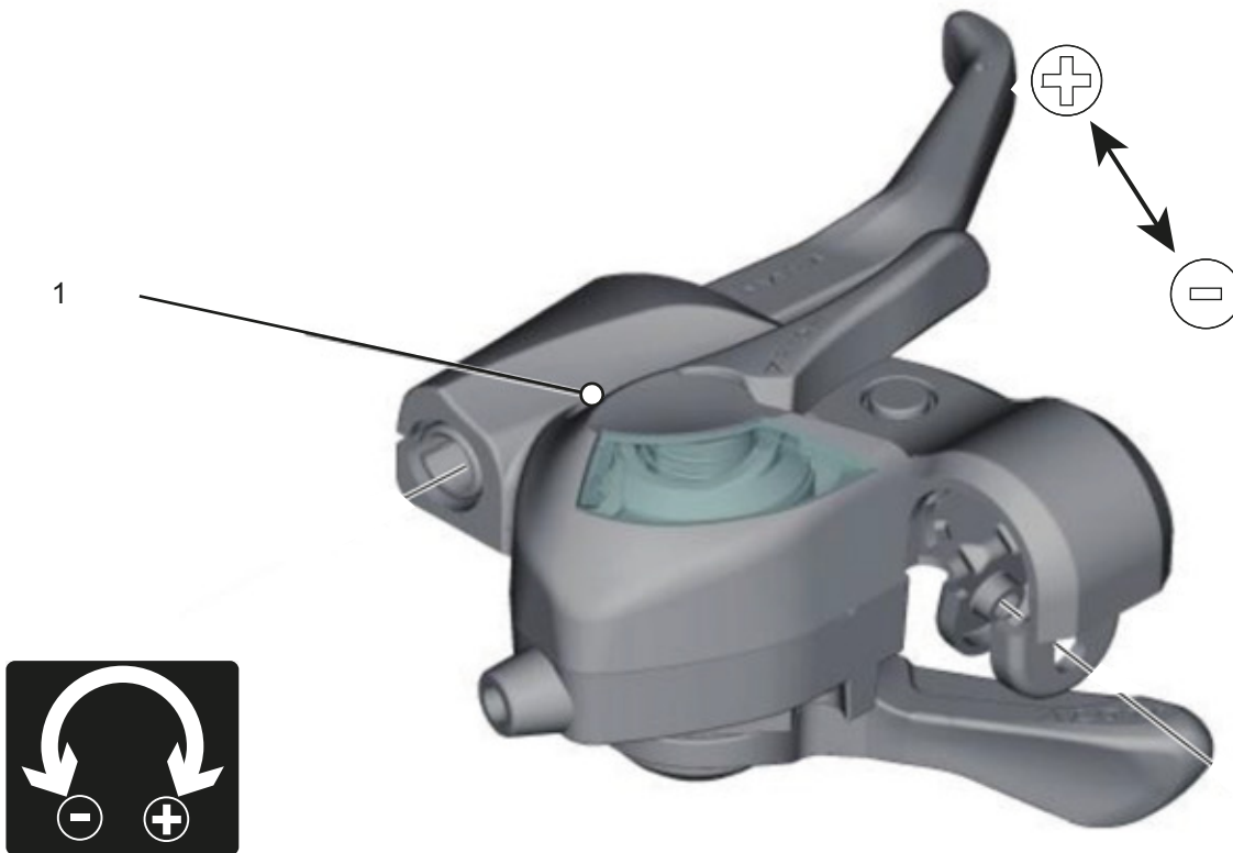
Figura 86: Posición del tornillo de ajuste (1)
