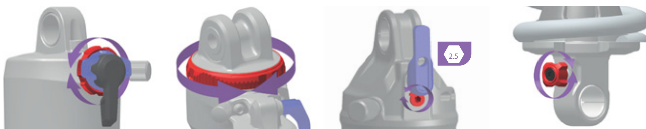
Figura 219: La posición y la forma del regulador de niveles de tracción (rojo) dependen del modelo
