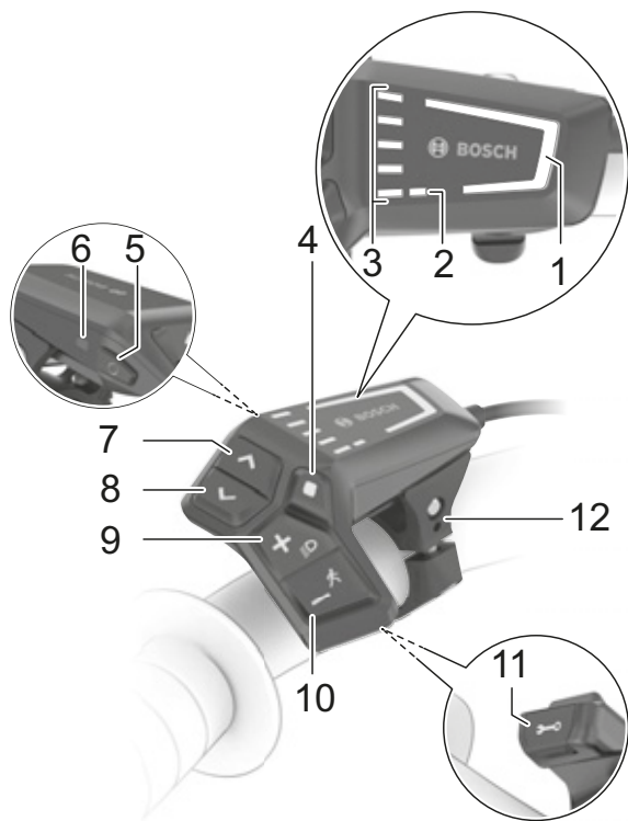
Figura 104: Vista general de la unidad de mando BOSCH LED Remote
