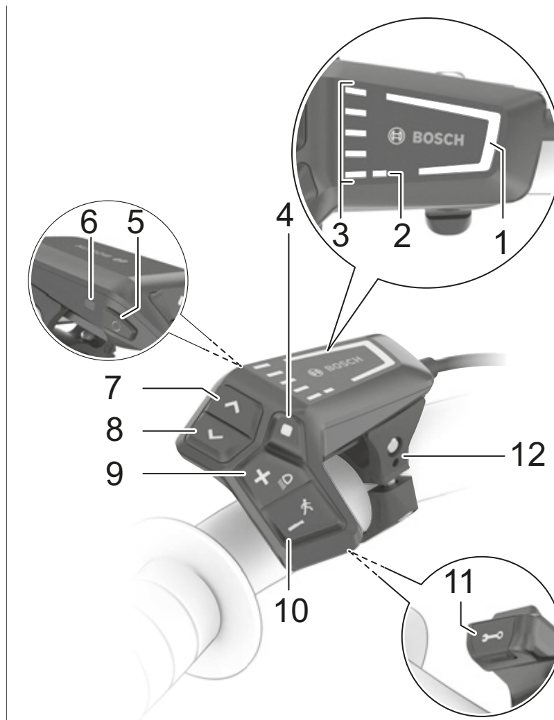
Figura 33: Vista general de la unidad de mando BOSCH LED Remote
