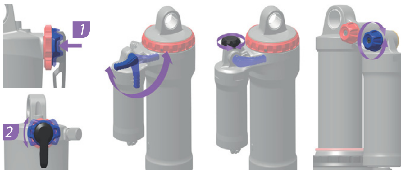
Figura 225: La posición y la forma del regulador de niveles de presión (azul) dependen del modelo
