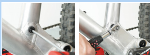
Figura 193: Atornillar la tija de sillín
