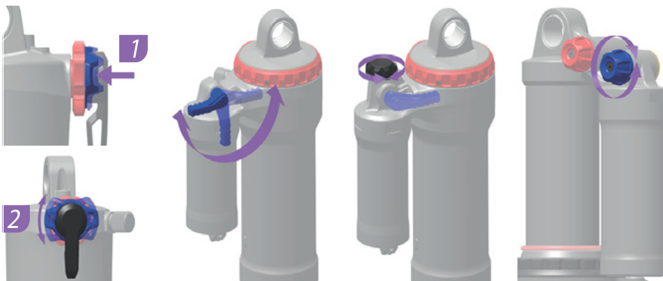
Figura 223: La posición y la forma del regulador de niveles de presión (azul) dependen del modelo
