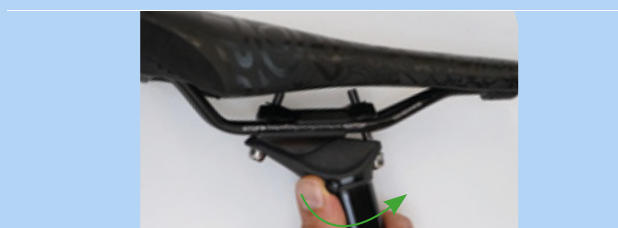
Figura 183: Apertura del ajuste de altura
